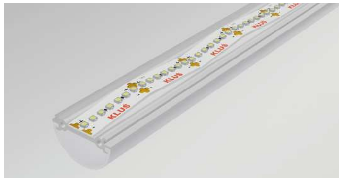
Faliste ułożenie taśmy może powodować nierówny rozsył światła. / Waves can cause uneven light distribution.
