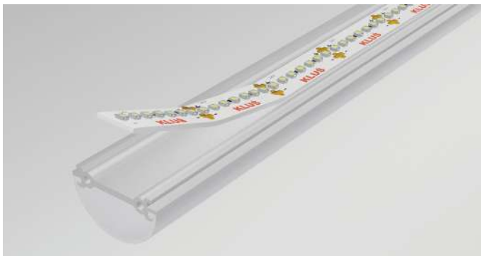
Po zdjęciu taśmy ochronnej wystarczy delikatnie docisnąć taśmę LED do powierzchni montażowej. / After removing the protective tape, just gently press the LED strip to the mounting surface.
